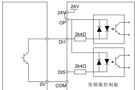
图 4-13 漏型接线方式内部供电示意图
