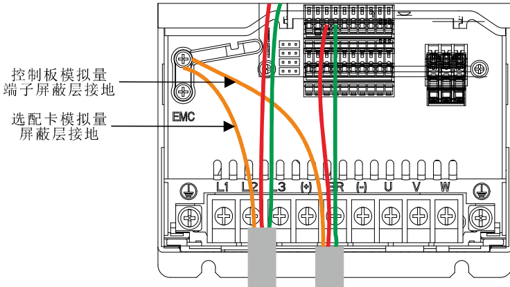
图 4-11 5K50G/7K50P~7K50G/11K0P模拟量端子的屏蔽层接地示意图
