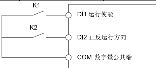
图 7-13 两线式模式2
