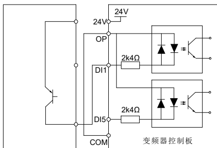
图 4-15 源型接线方式内部供电示意图
