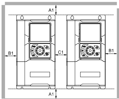
图 3-7 变频器安装空间（并列多台安装）
