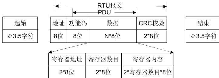
图 1 RTU 模式报文帧示意图
