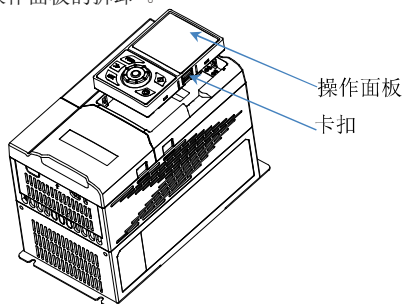
图4-2 变频器操作面板的拆卸
