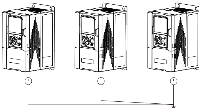
图 4-7 接地方式
