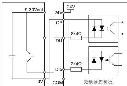
图 4-14 源型接线方式外部供电示意图
