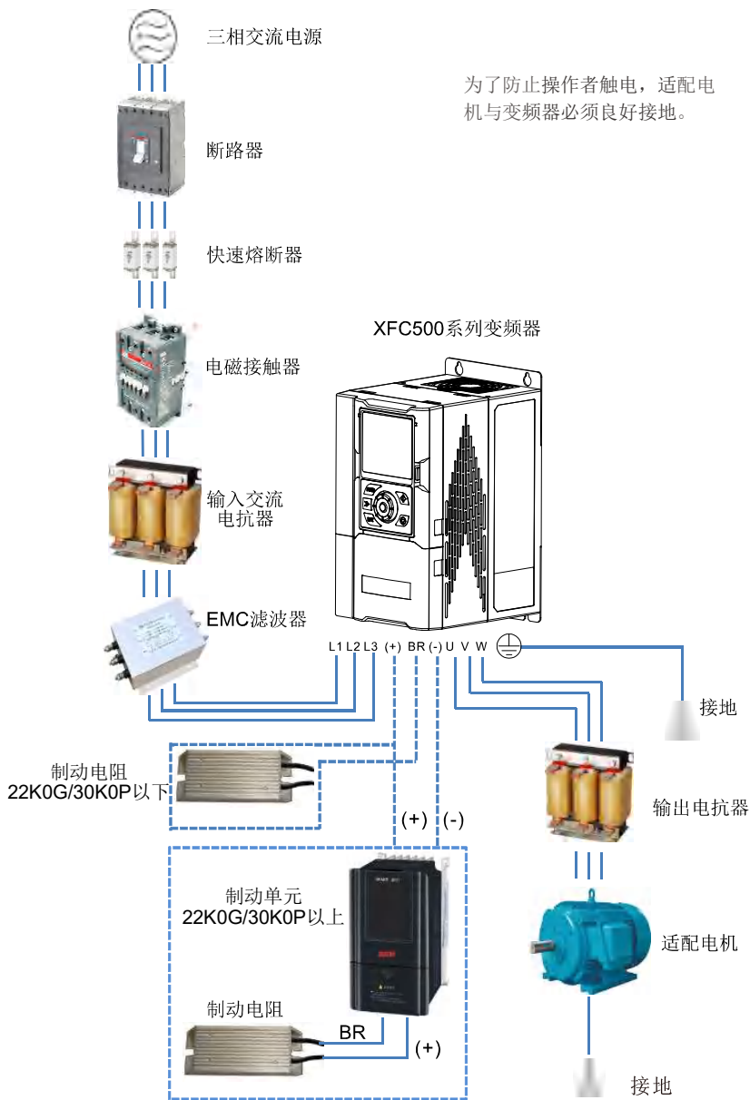
图 2-3 系统外围配线
