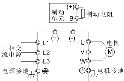
图 10-4 30K0G/37K0P以上机型接制动电阻
