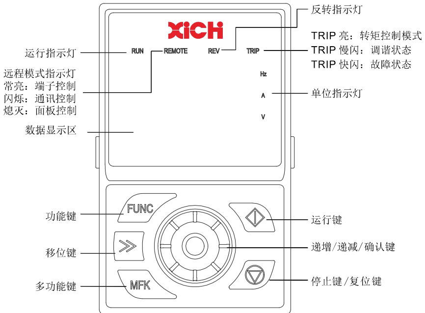
图 5-1 操作面板各部分名称与功能
