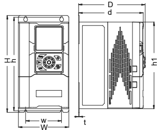
图 3-2 变频器外形图B
