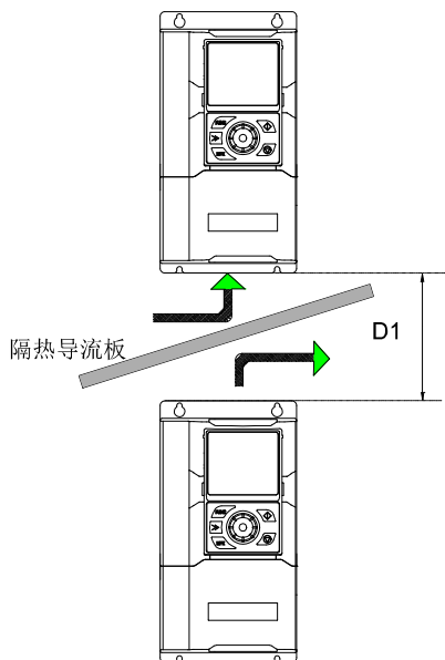
图 3-8 变频器安装空间（上下安装）
