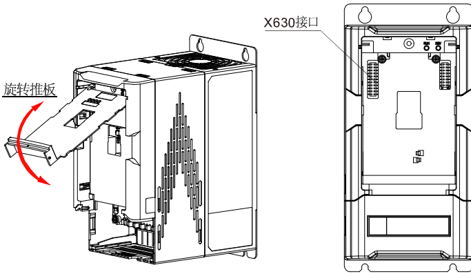
图 10-2 扩展卡的安装
