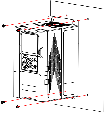
图 3-9 变频器壁挂式安装
