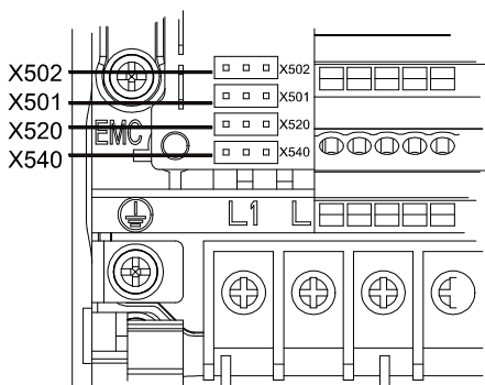
图 4-18 X502/X501/X520/X540位置所在图
