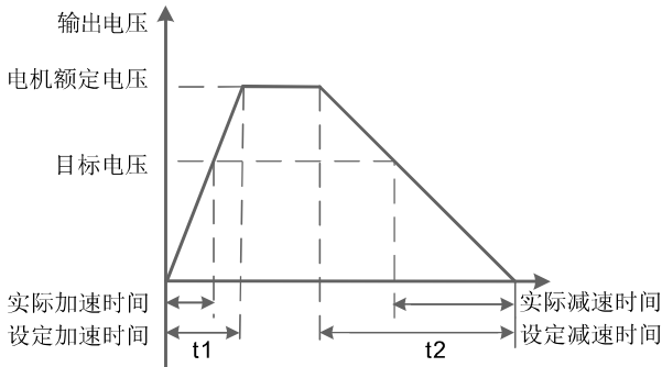
图 7-4 V/F分离示意图
