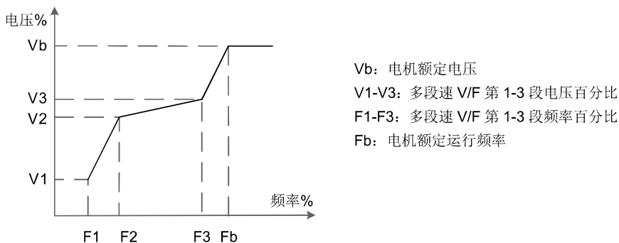
图 7-3 多点V/F曲线设定示意图
