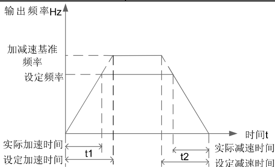
图 7-8 加减速时间示意图
