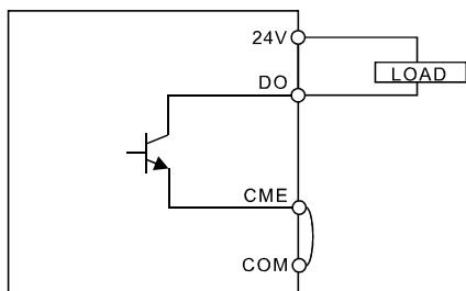
图 4-16 数字输出端子内部供电接线示意图
