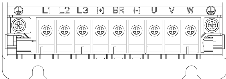
图 4-6 主回路端子分布示意图
