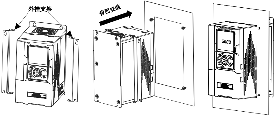
图 3-10 塑胶结构嵌入式安装步骤图
