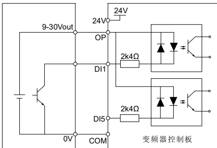
图 4-12 漏型接线方式外部供电示意图
