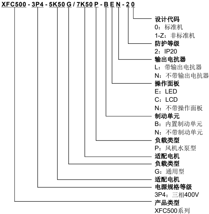
图 2-1 变频器型号说明
