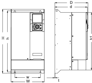
图 3-3 变频器外形图C
