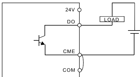
图 4-17 源数字输出端子外部供电接线示意图
