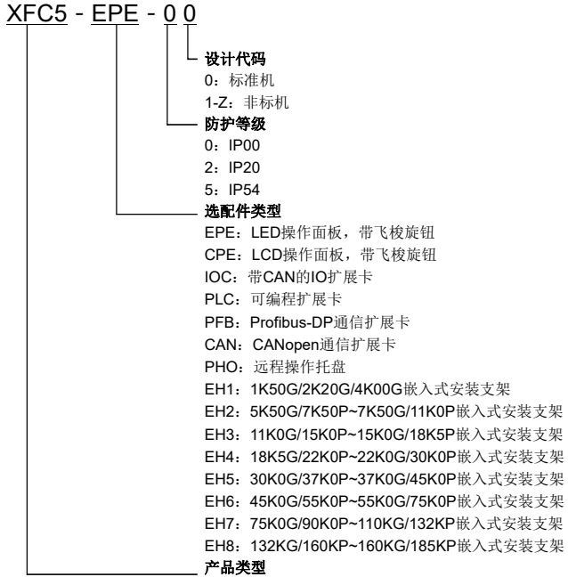
图 10-1 选配件类型编码说明
