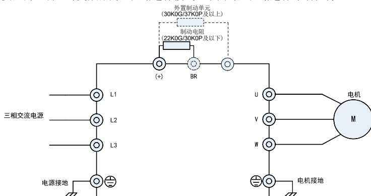
图 4-5 主回路连接图
